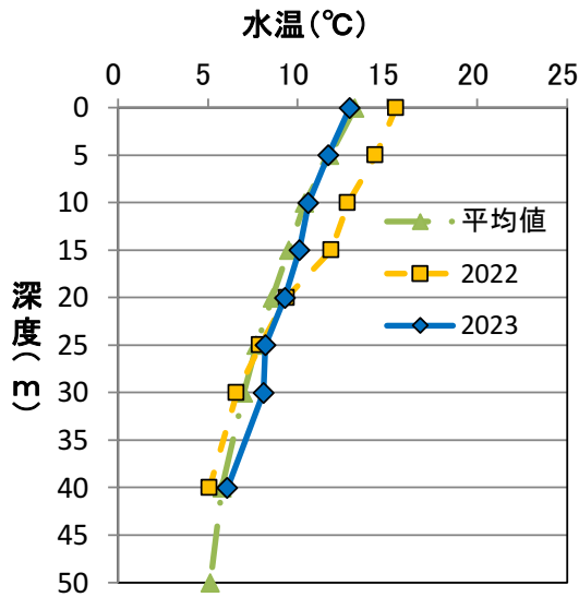
水温の鉛直分布
