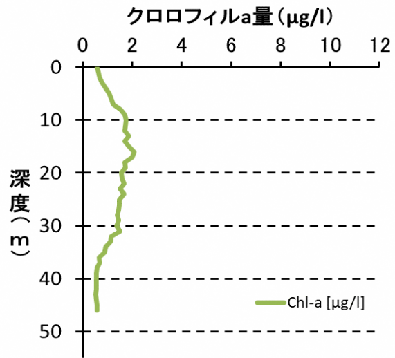
クロロフィルa量の鉛直分布
