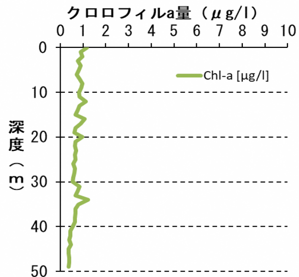
クロロフィルa量の鉛直分布
